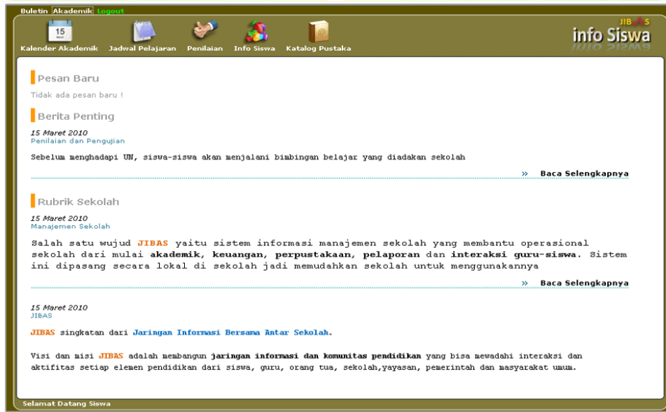
Gambar 19. Menu Akademik
